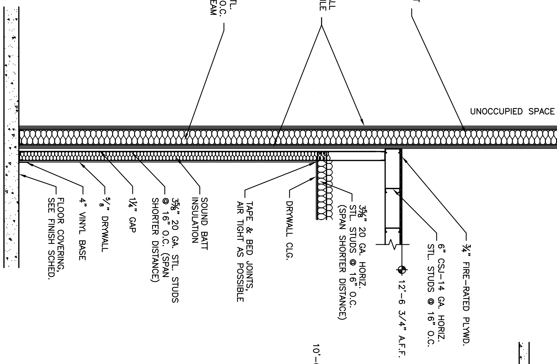
SECTION 10 SCALE: 1/2" = 1'-0"
